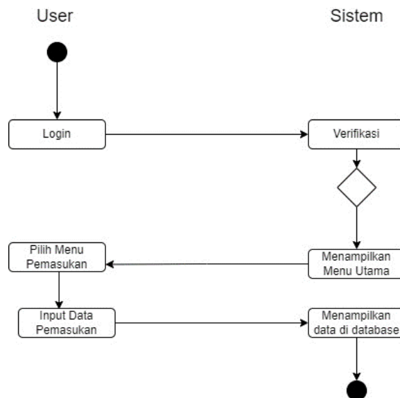
Gambar 3. 3 Diagram Activity Menu Pemasukan
