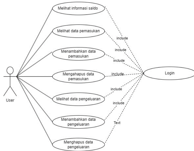
Gambar 3. 2 Use case diagram aplikasi pengelolaan keuangan
