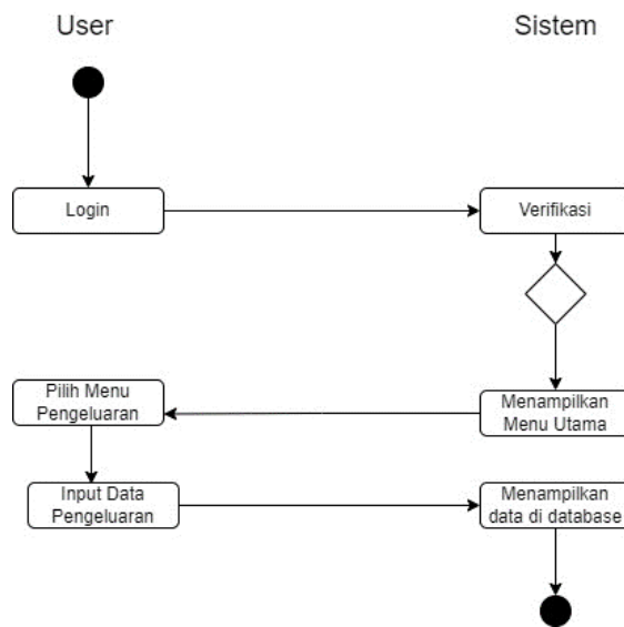
Gambar 3. 4 Diagram Activity Menu Pengeluaran
